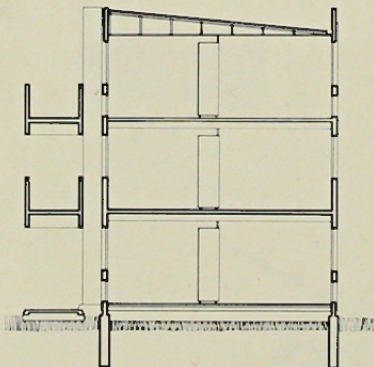
CORTE
