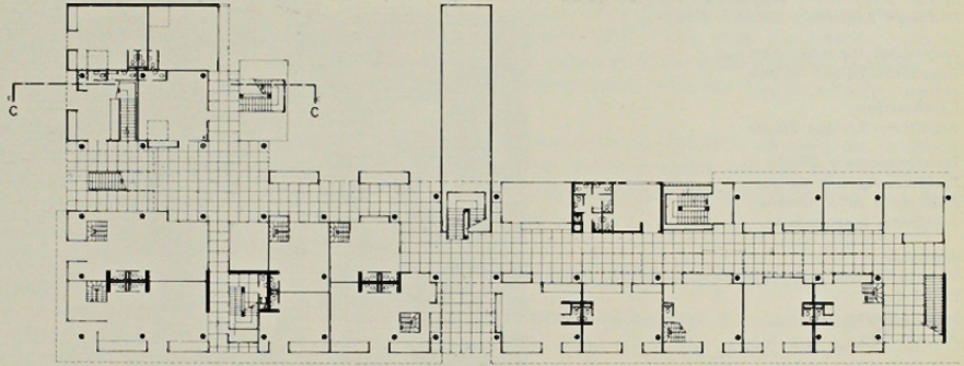
PLANTA 1º PISO
