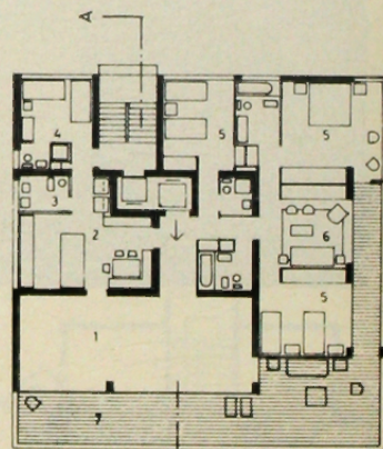
PISO TIPO
