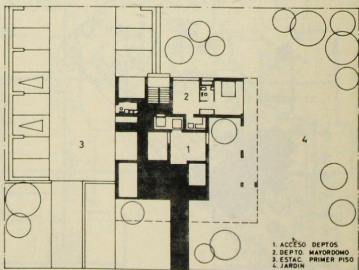
PLANTA GENERAL
